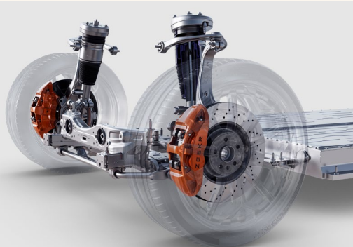
דיסקי בלם מאווררים מתוצרת Brembo, בשילוב קאליפרים בעלי 4 בוכנות מתוצרת Continental *ברמת גימור Krypton בלבד
