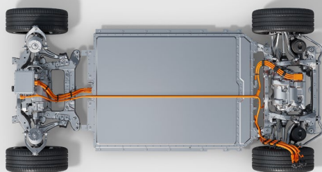
ארכיטקטורה 800V
