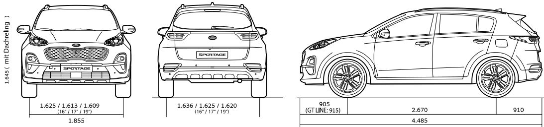
מידות (מ"מ)
